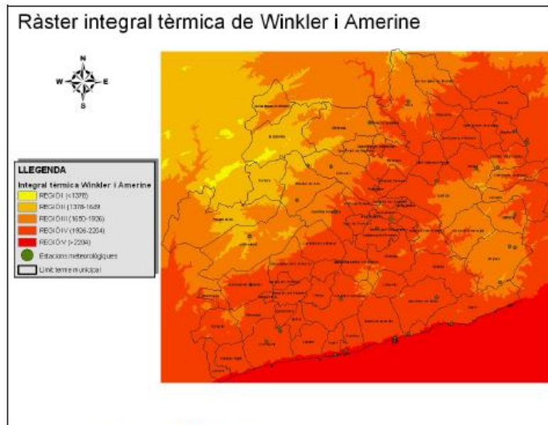
Figura 4: Ràster integral tèrmica Winkler i Amerine.
